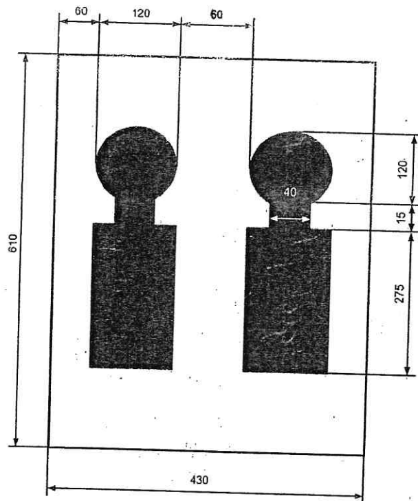
Rysunek 4-1. Tarcza T1 (strefa trafień skutecznych).
