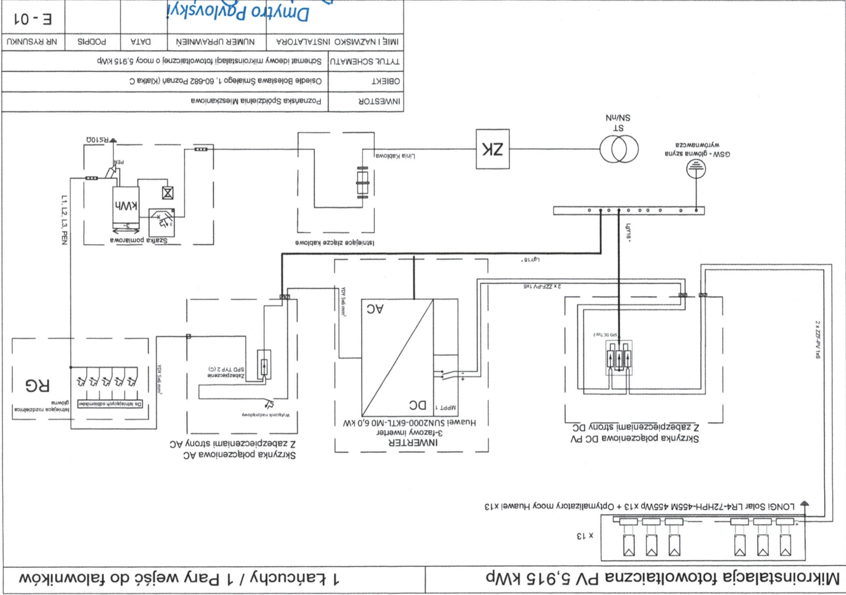
Schemat elektryczny mikroinstalacji fotowoltaicznej o mocy 5,915 kWp (klatka C)
