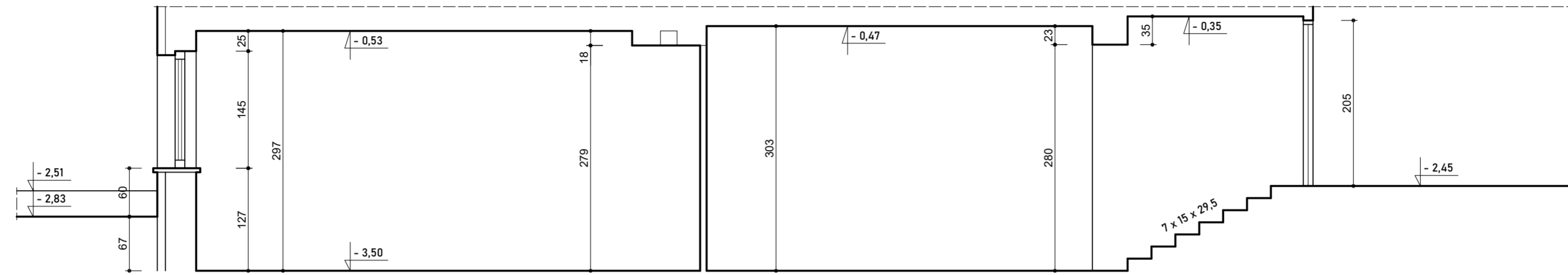
Przekrój A - A
