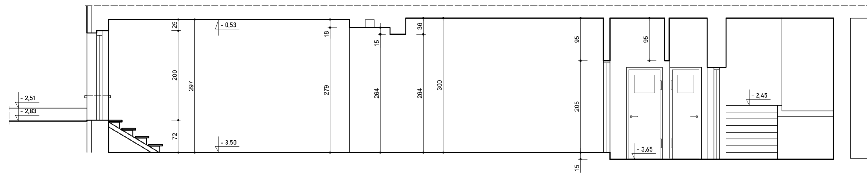
Przekrój B - B
