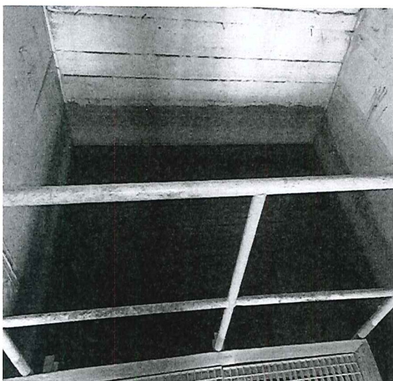
Zbiorniki ścieków oczyszczonych zlokalizowane przy oczyszczalni (miejsce zabudowy pomp ścieków)
