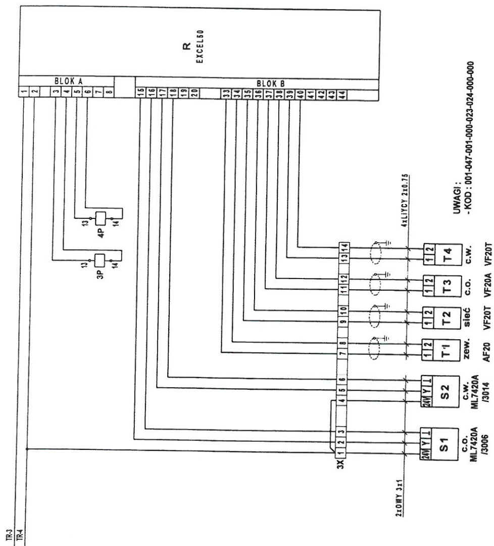
Schemat ideowo-montażowy instalacji elektrycznej węzła typu ECWS-500/300 (regulator temperatury)
