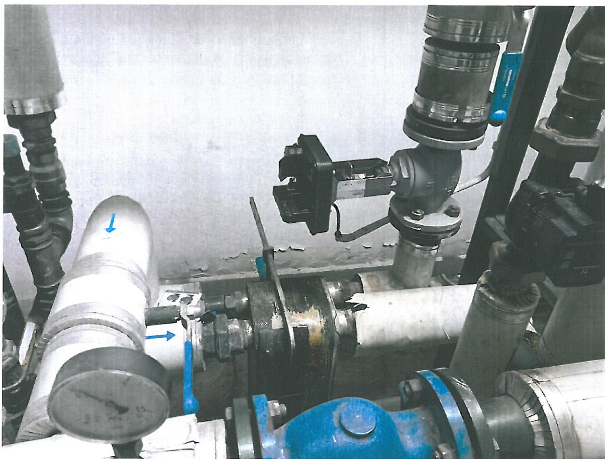
Fot.2 – Stacja wymienników ciepła – WIDOK GŁÓWNYCH USZKODZEŃ
