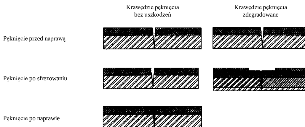
Rys. 2. Wypełnienie pęknięcia poszerzonego przez frezowanie
