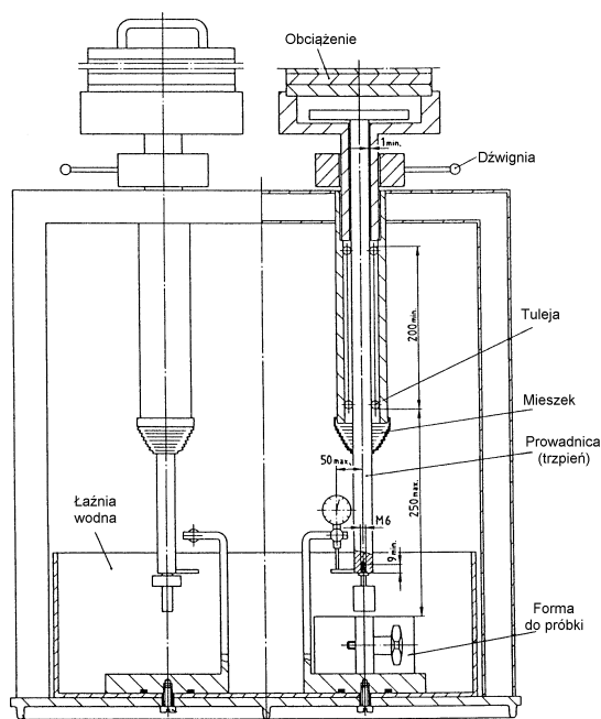
Rys. 2. Stempel penetrometru
