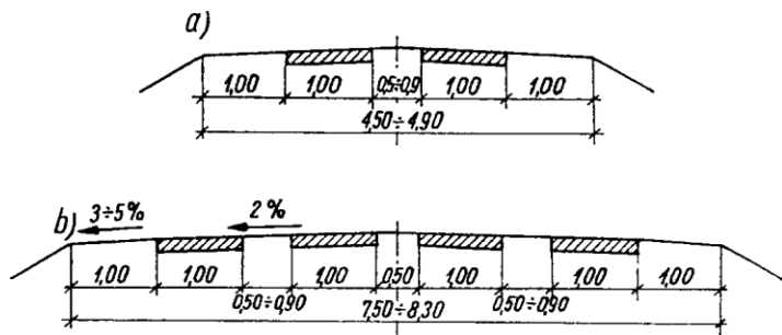
Rys. 5. Układanie płyt na łuku o małym promieniu
