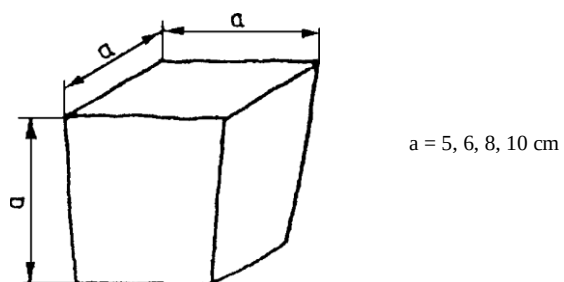
Rys. 2. Desenie chodnika z kostki kamiennej nieregularnej
