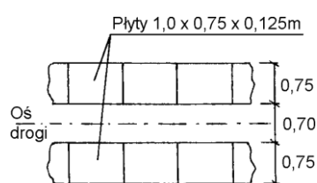
Rys. 2. Przykłady ułożenia płyt na jezdni jednopasowej
