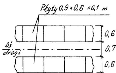
Rys. 2. Przykłady ułożenia płyt na jezdni jednopasowej
