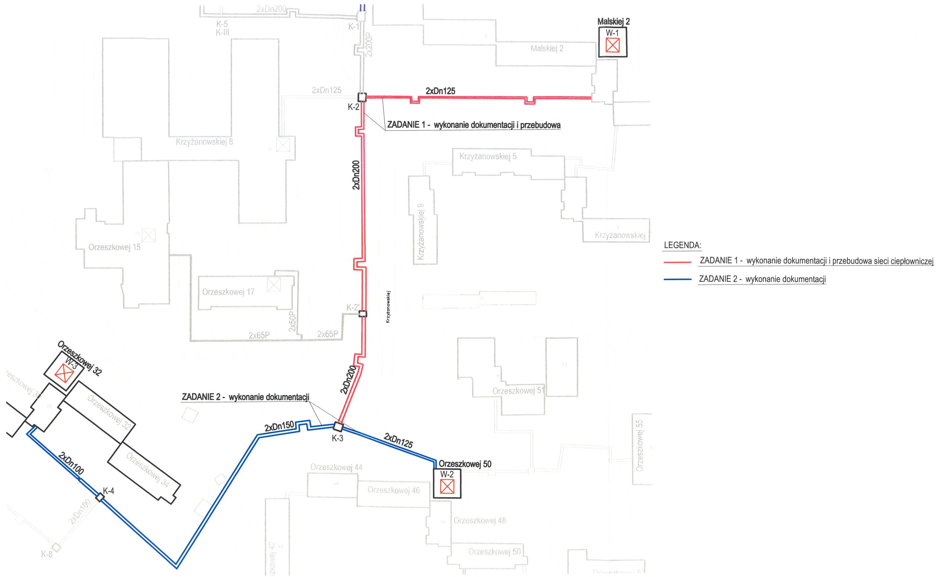
Załącznik nr 1 c - Załącznik graficzny z zakresem przebudowy sieci ciepłowniczej i zakresem dokumentacji projektowej
