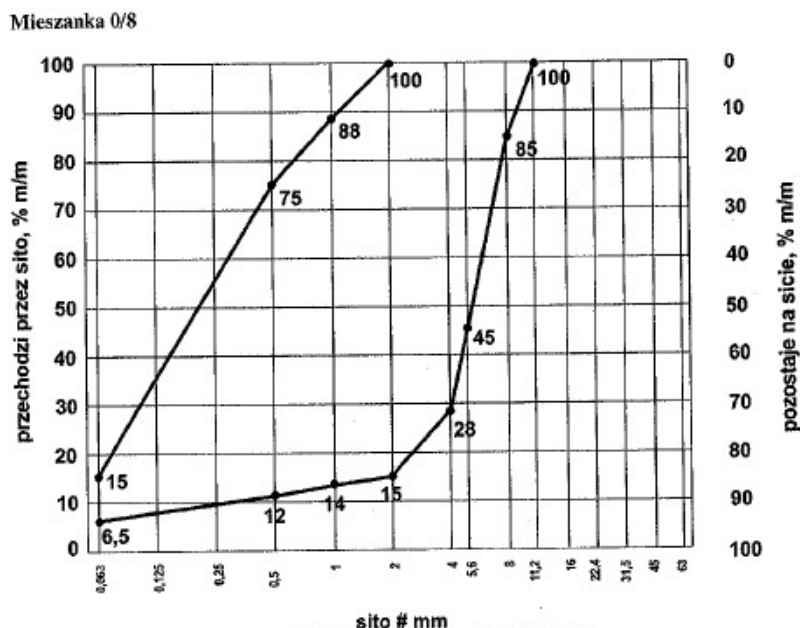
Rys. 1.5. Uziarnienie mieszanki CBGM 0/8
